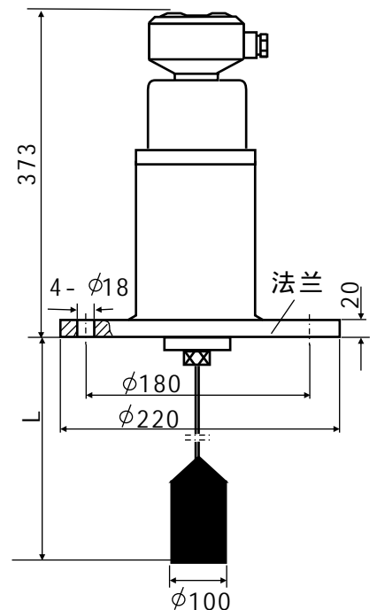
图三 重型缆式探极
