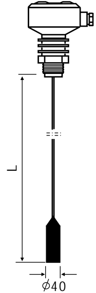
图四 轻型缆式探极
